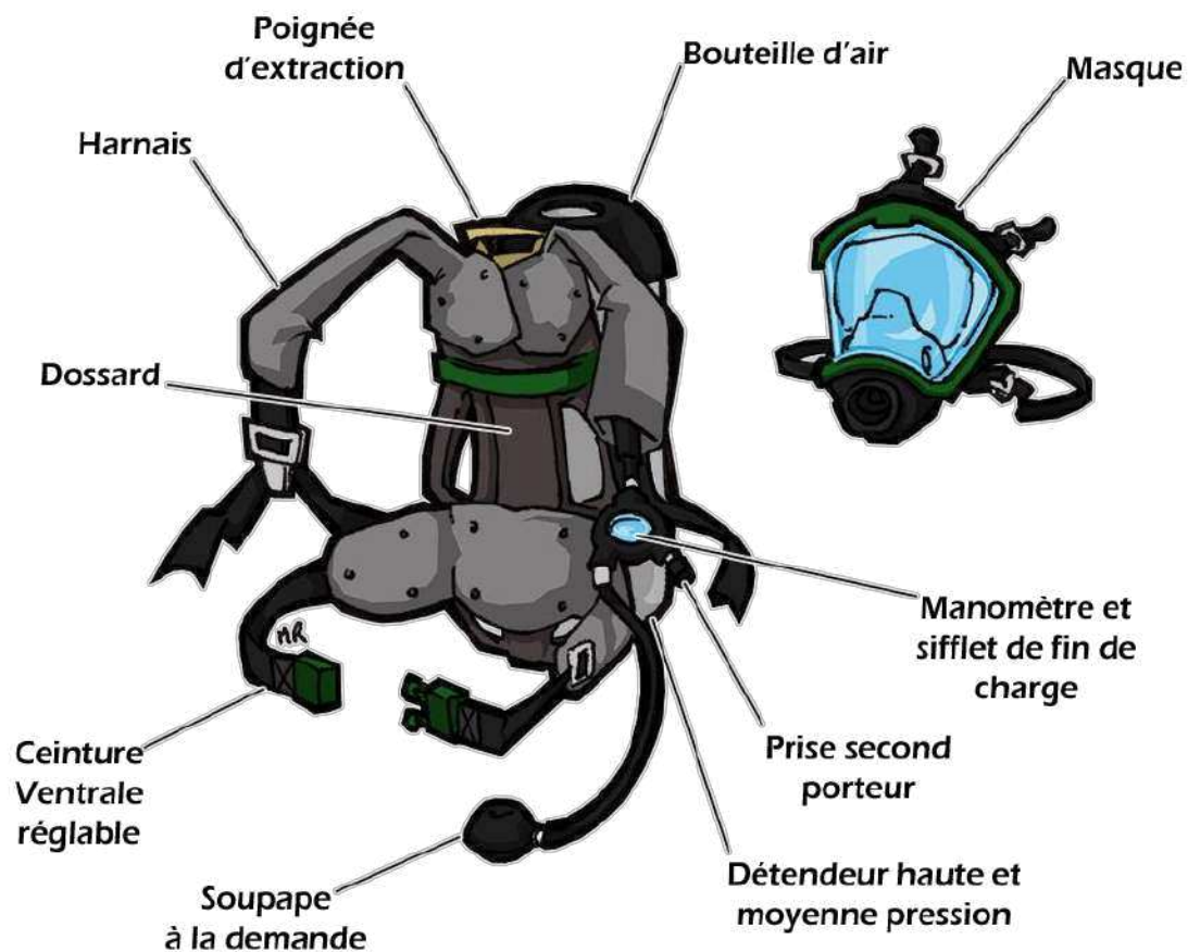
Schéma de principe d'un appareil respiratoire isolant à circuit ouvert
